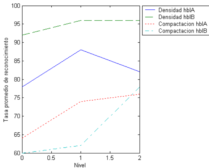
Fig. 7.1: Tasas de reconocimiento para vocales.
