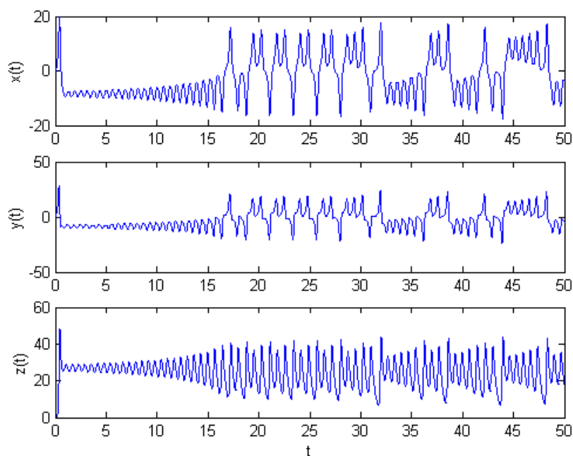
Fig. 2.5: Series de tiempo caóticas generadas por las ecuaciones de Lorenz.
