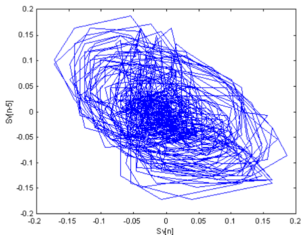
Fig. 2.7: Espacio de Fase Reconstruido a partir de una señal verbal arbitraria, con m = 2 y \tau = 5 .
