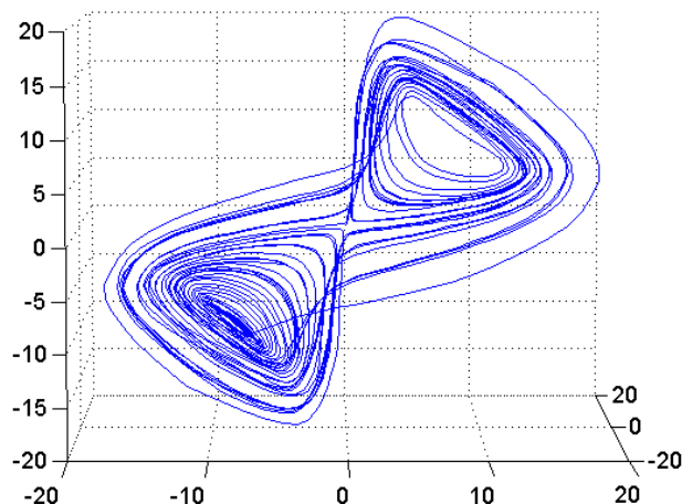
Fig. 2.8: Espacio de Fase Reconstruido a partir de x(t) en las ecuaciones de Lorenz, con m = 3 y \tau = 6 .
