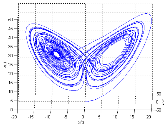
Fig. 2.6: Espacio de Fase tridimensional con el atractor de Lorenz.
