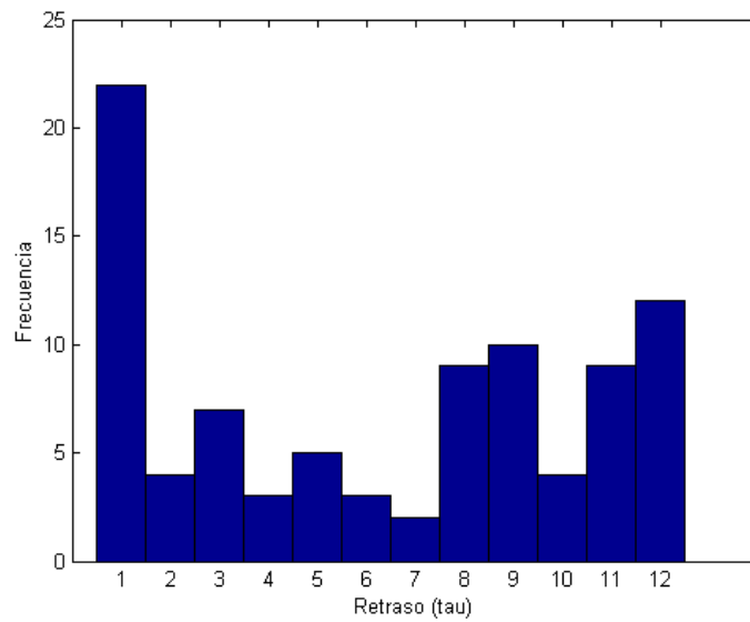
Fig. 5.4: Histograma combinado del retraso ( \tau ) en la reconstrucción de las señales en C_E^V .
