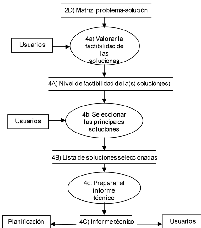
Figura 5. Diagrama de flujo de datos expandido del proceso 4. Fuente: Jaimes et al. (2007).
