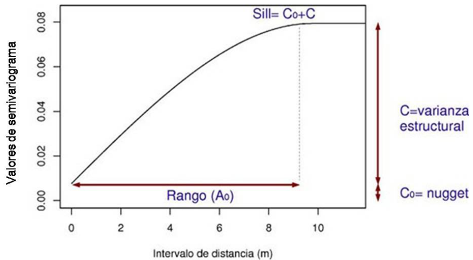
Figura 3.5 Esquema de un semivariograma y valores que se extraen ( C_0 , C_0+C , A_0 ) a partir del modelo matemático que mejor se ajuste. La curva representa el modelo matemático que mejor se ajusta a la dispersión de puntos antes de alcanzar la meseta.
