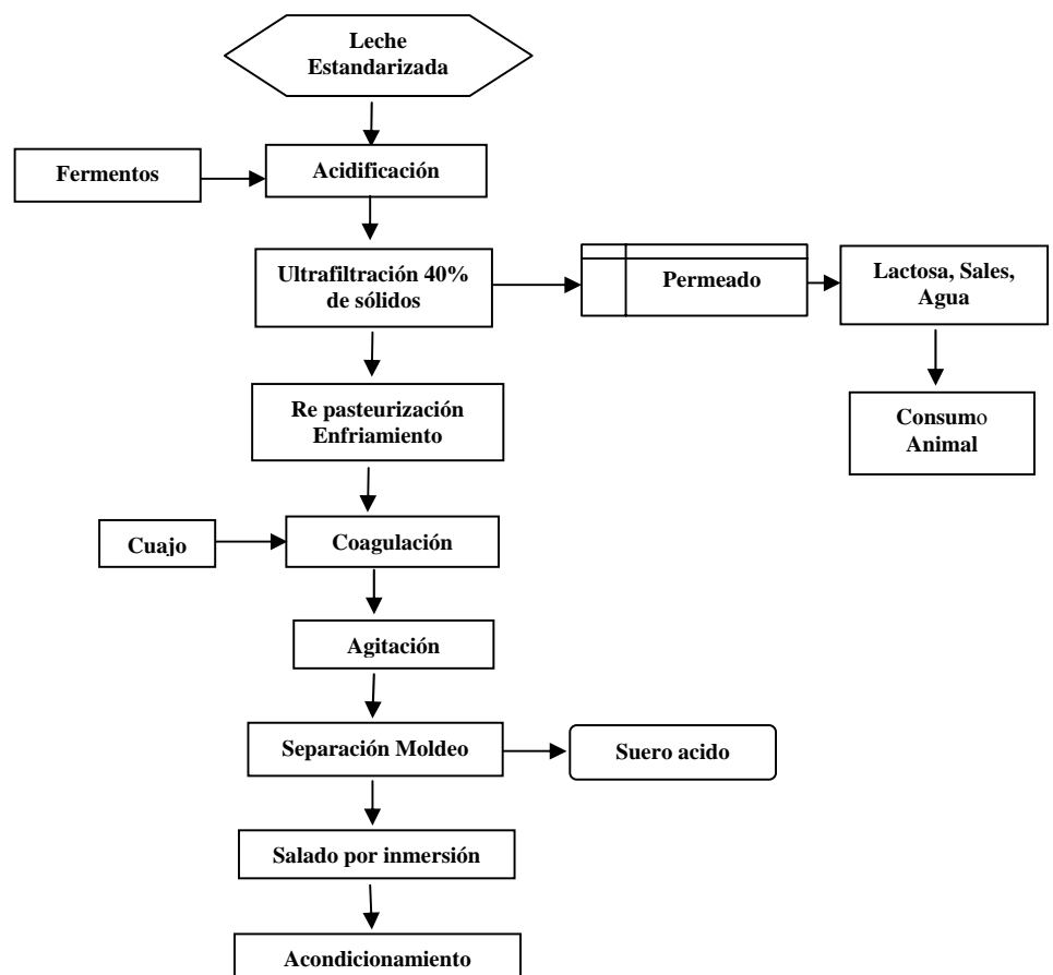
Figura 3. Flujograma de elaboración de queso blanco por tecnología de UF.
