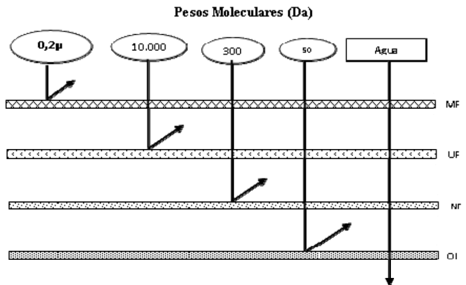
Figura 2. Características de los procesos de membrana.
