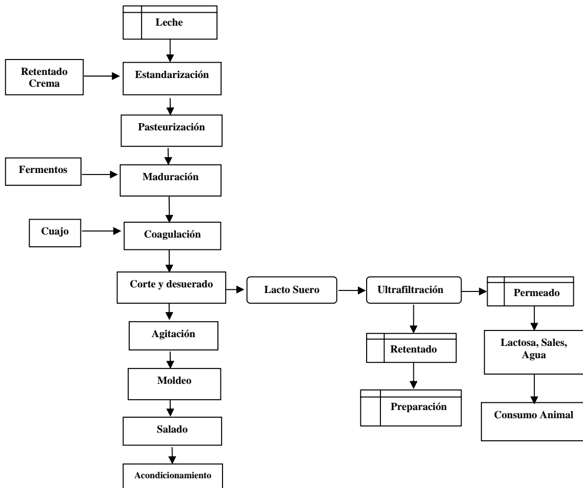
Figura 4. Flujograma de elaboración de queso PE con incorporación de proteínas.
