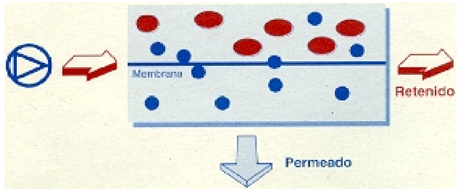
Figura 1. Esquema de separación por Filtración Tangencial.
